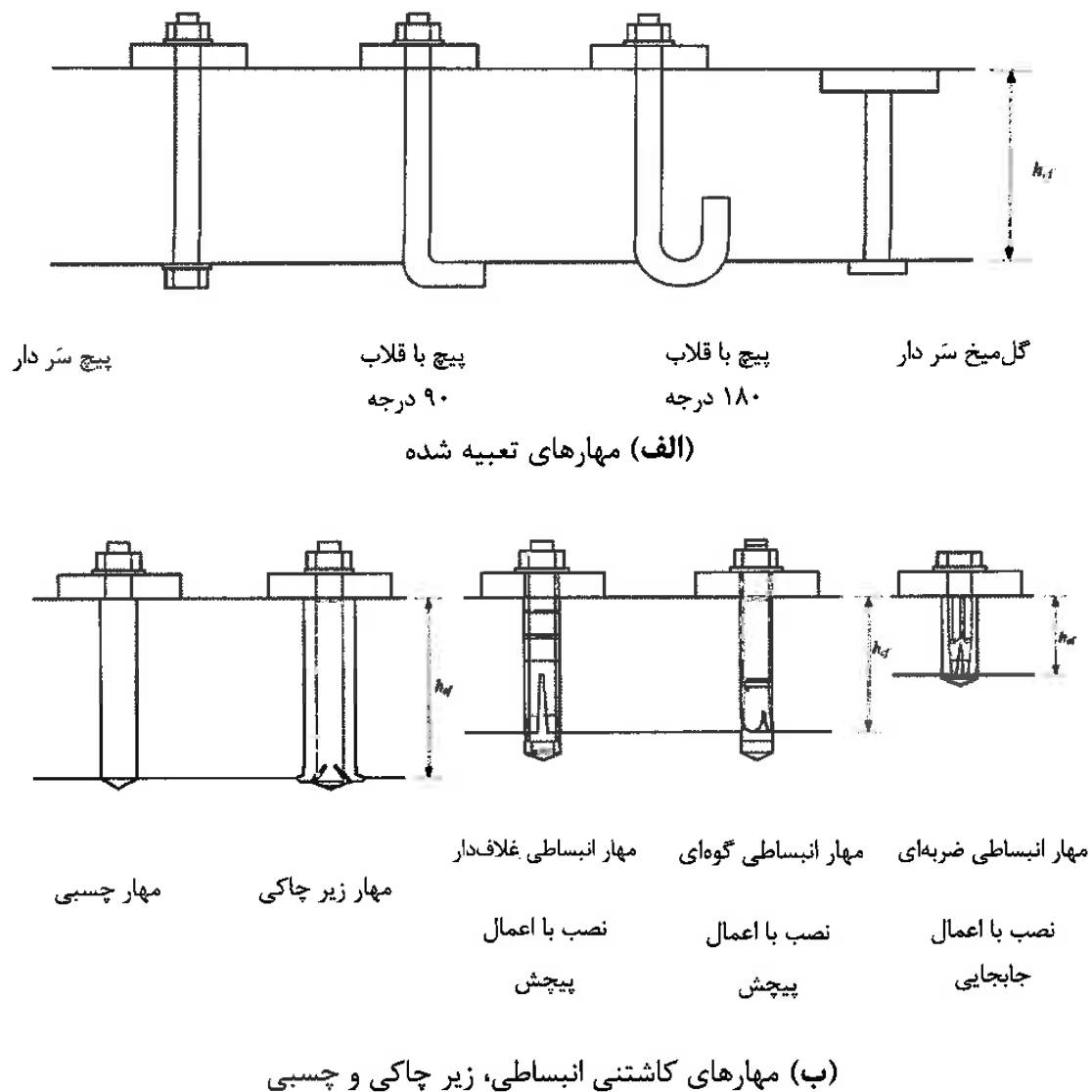
شکل ۹-۱۸-۱ انواع مهارها
