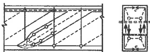
پ- عضو فشاری قطری درجهان فارای خلعت
