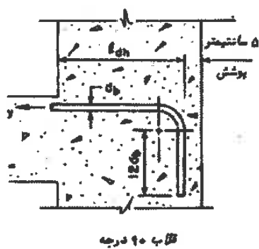
شکل ۹-۵ پ-۵ چگونگی اتصال تیر به ستون در گوشه
